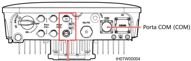
Terminali della batteria (BAT+/BAT-)
